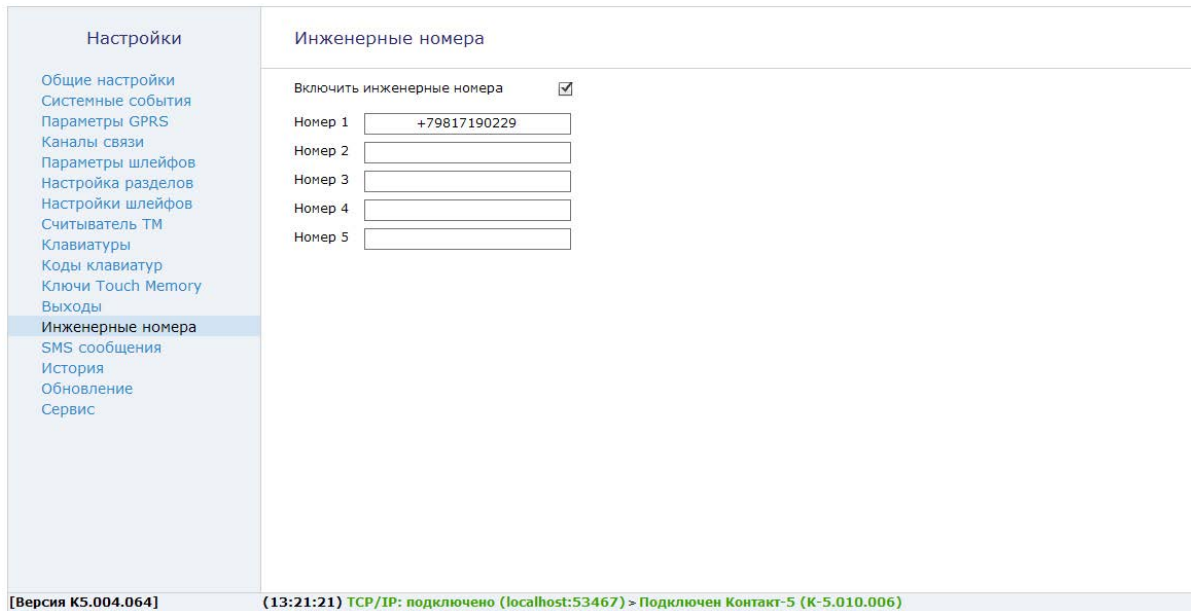
Рисунок 30. Раздел «Инженерные номера»
