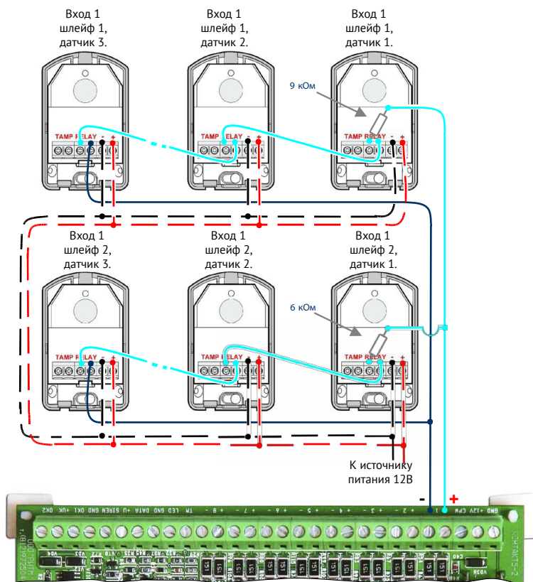
Рисунок 38. Схема подключения охранных датчиков на вход №1
