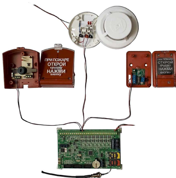
Рисунок 45. Фотография подключения пожарных датчиков
