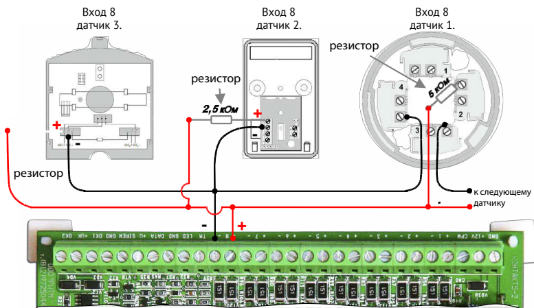
Рисунок 43. Схема подключения пожарных датчиков на вход №8
