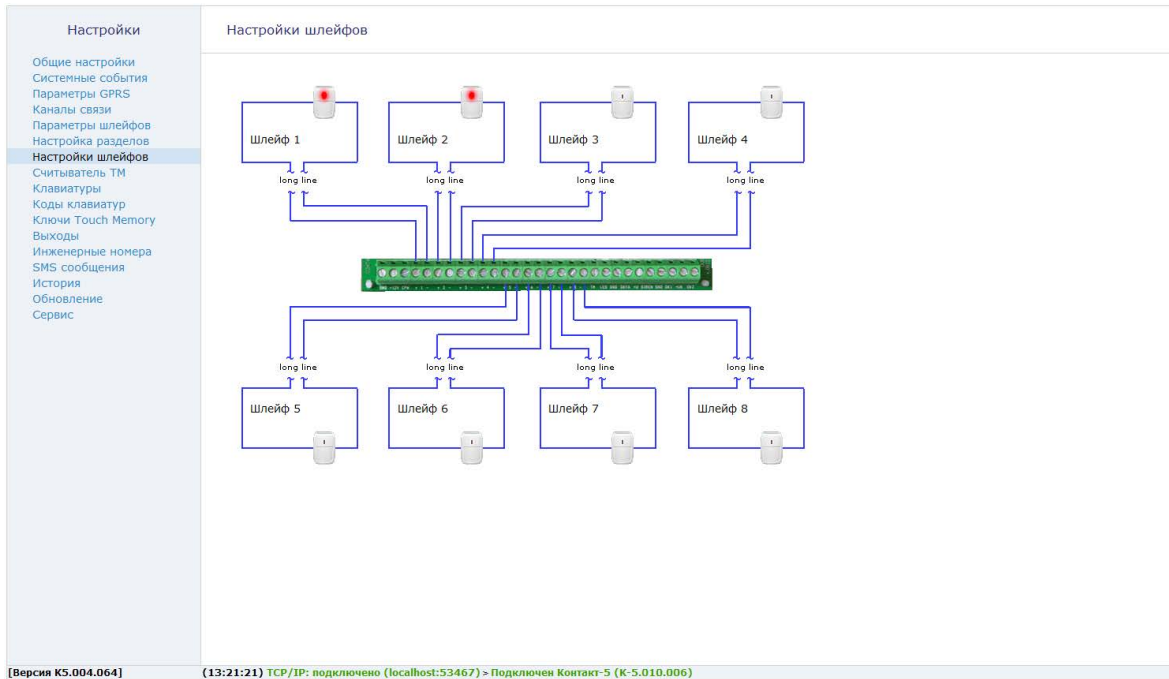
Рисунок 20. Настройки шлейфов: шлейфы типа «сухой контакт»
